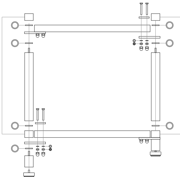
MODULAR RACK RS2 /CODE - MR-RS2/
